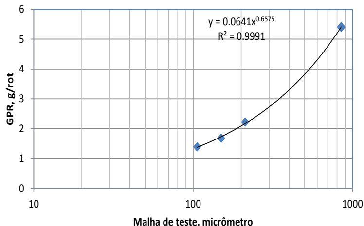
Figura 2. Correlação entre a malha de teste e o valor de GPR para a amostra de minério de titânio.
