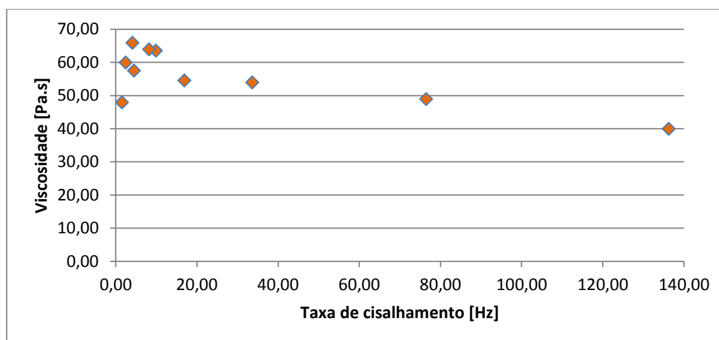
Figura 6. Viscosidade versus taxa de cisalhamento para o sebo bovino a 60° C.
